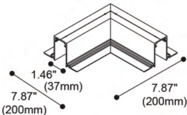
Moduel d'angle horizontal
