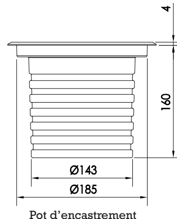
Pot d'encastrement
